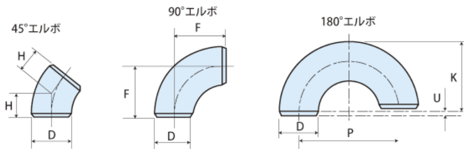
45°エルボ,90°エルボ及び180°エルボの形状・寸法
