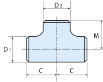
同径Tの形状・寸法
